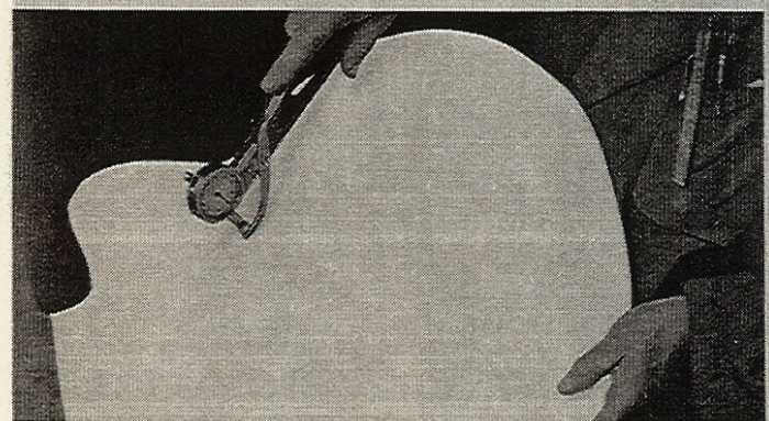
Mätning av locket's tjocklek
