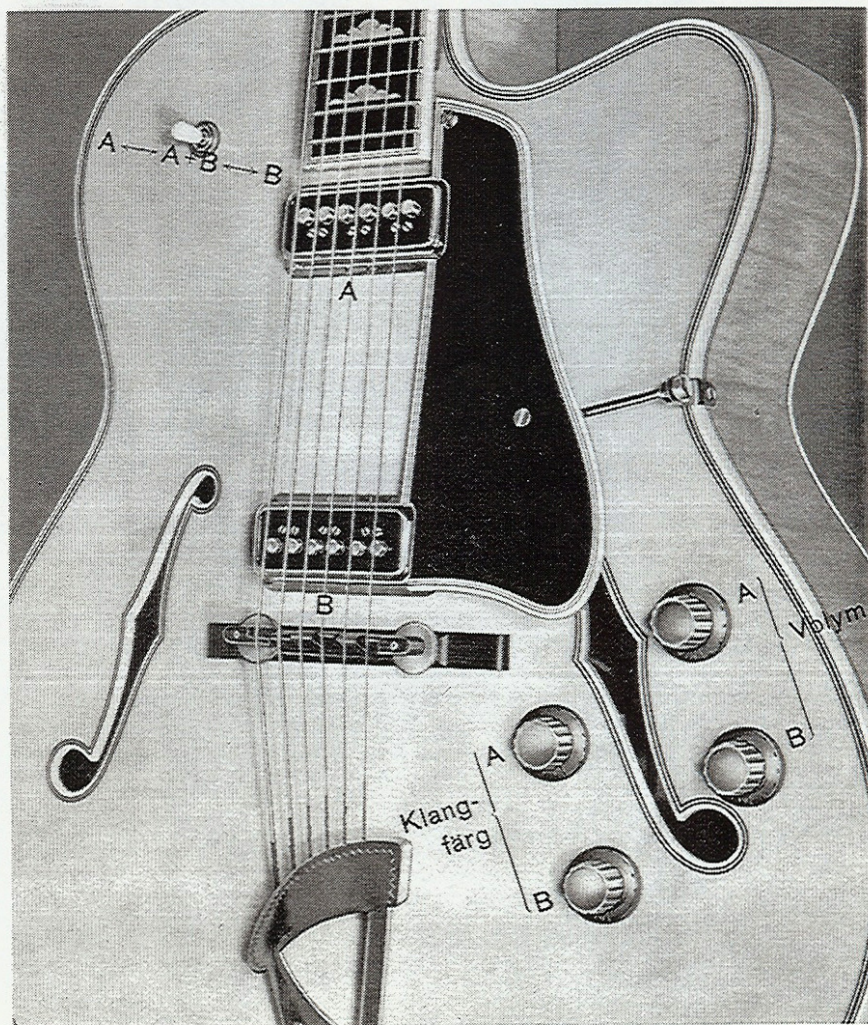
Gitarr nr 315N/M2. Längst upp till vänster mikrofonväljare med tre olika lägen (enbart mikrofon A, båda mikrofonerna, enbart mikrofon B).
